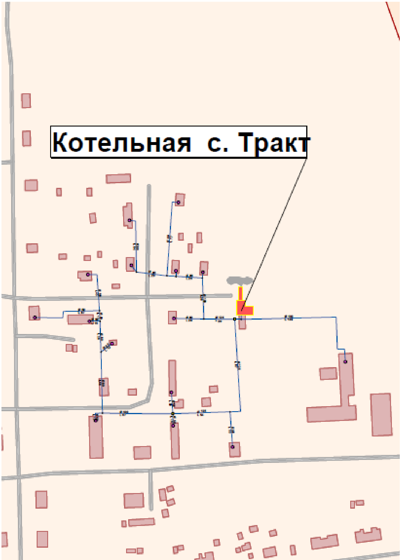
Рисунок 2.1 – Схема тепловых сетей
