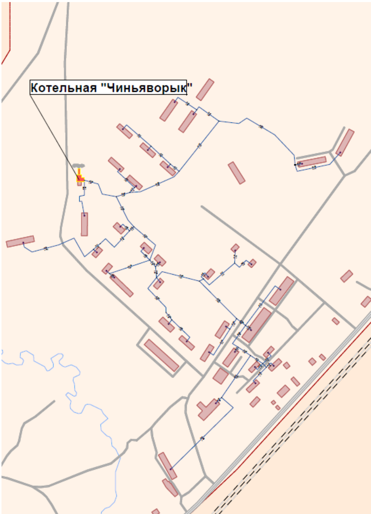
Рисунок 2.1 – Зона действия котельной с. Чиньяворык.
